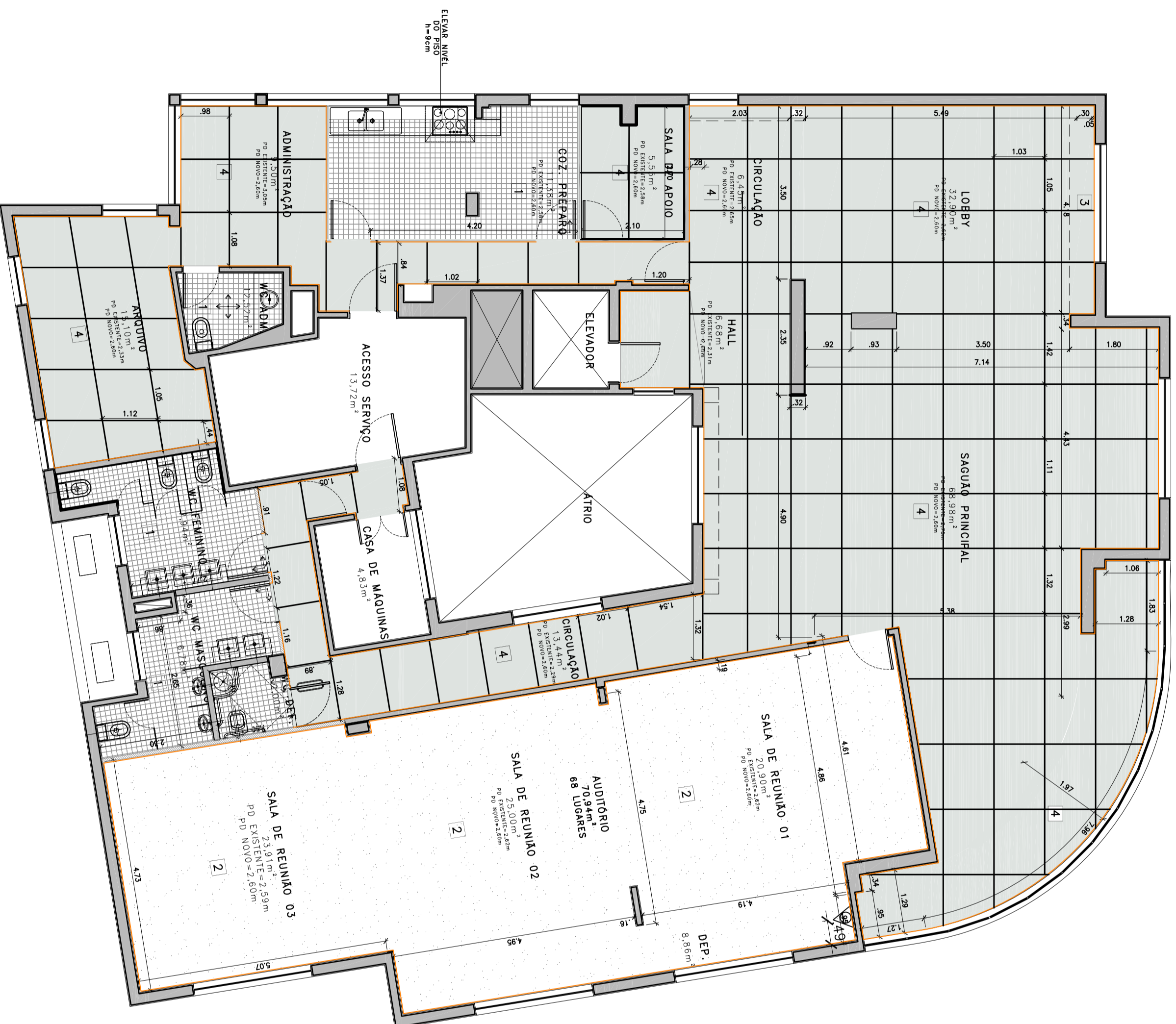
PLANTA DE PISO ESC: 1:75
